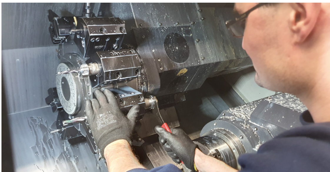
Die Abstandhalter sind aus Edelstahl und werden vorrangig mit Dreh- und Frästechnik hergestellt.
